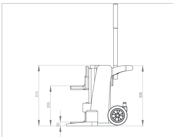
JH 15 G plus EX | Art-No. 11 615 106-G | Seitenansicht | Side view
