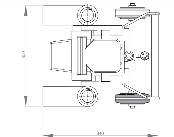
JH 15 G plus EX | Art-No. 11 615 106-G | Draufsicht | Top view
