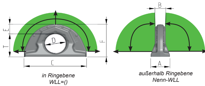
Abb. 5: Bemaßung - zulässige Belastungsrichtungen
