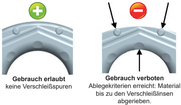
Abb. 3: Verschleißmarkierungen
