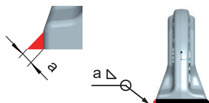
Abb. 4: Schweißnahtanordnung
