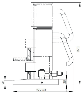
JHS 10 ku | Art.No. 01 020 10S-O | Seitenansicht | Side view
