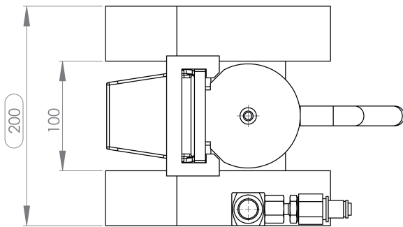
JHS 10 KU | Art.No. 01 020 105-O | Draufsicht | Top view
