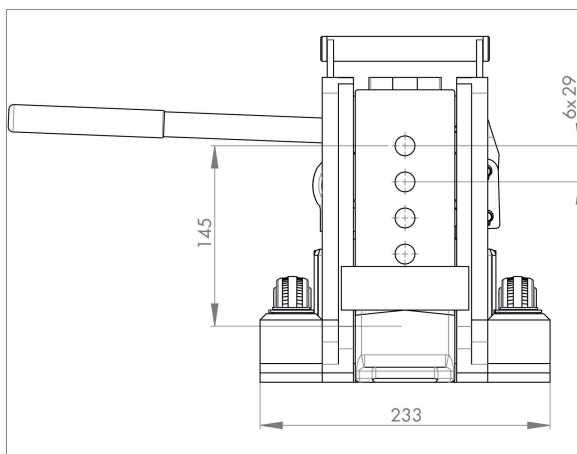
JH 6 G plus | Art.No. 01 060 102-G | Seitenansicht | Side view
