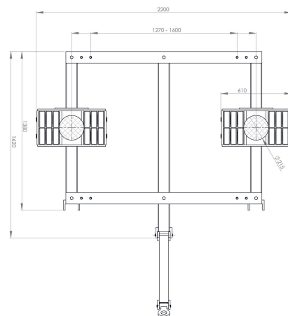
JTLB 30 G | Art.No. 12 302 140-V2 | Draufsicht | Top view
