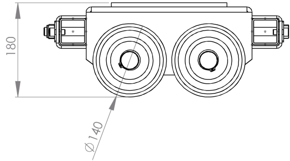
JFB 30 G | Art-No. 10 302 140-V | Seitensicht | Side view
