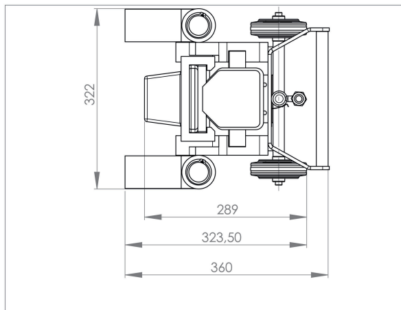
JH 20 G plus EX | Art-No. 11 620 106-G | Draufsicht | Top view
