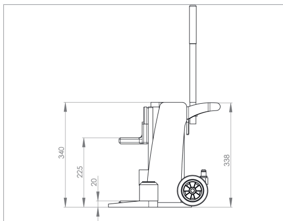
JH 20 G plus EX | Art-No. 11 620 106-G | Seitenansicht | Side view
