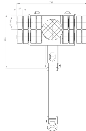
JLB 20 G | Art-No. 09 202 140-V | Draufsicht | Top view
