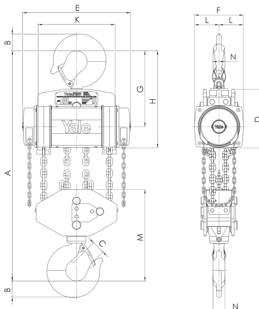
Yalelift 360, 20.000 kg, sechssträngig
