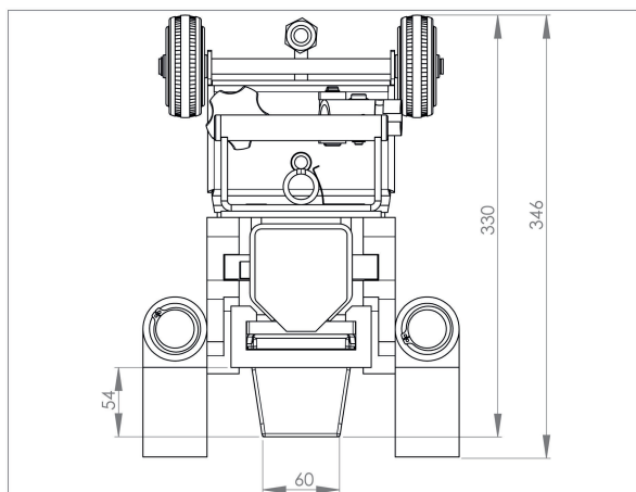
JH 10 G plus | Art-No. 01 100 102-G | Draufsicht | Top view
