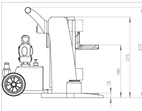
JH 10 G plus | Art-No. 01 100 102-G | Seitenansicht | Side view
