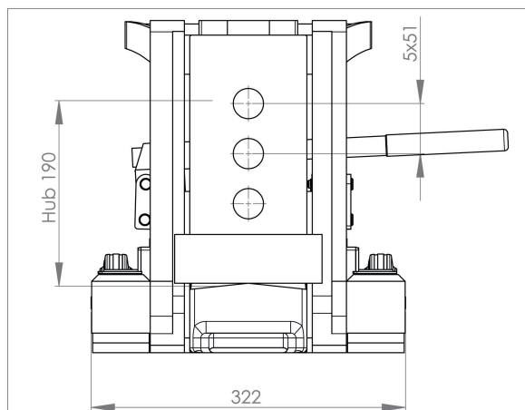
JH 20 G plus | Art.No. 01.200.102-G | Frontansicht | Front view
