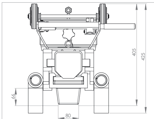
JH 20 G plus | Art.No. 01.200.102-G | Draufsicht | Top view
