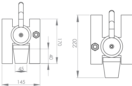
Lasche abgestützt / Supported toe
