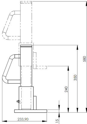
JHS 5 | Art.No. 01 020 050-O | Seitenansicht | Side view
