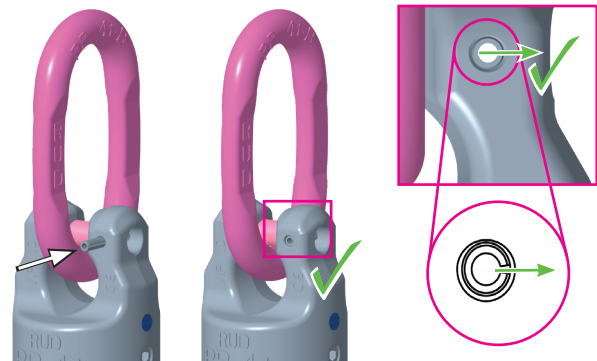
Abb. 4: Montage Spannstift
