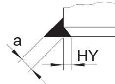
Abb. 9: Schweißnahtanordnung
