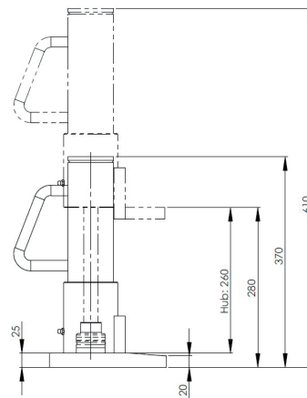
JHS 10 | Art.No. 01 020 101-O | Seitenansicht | Side view
